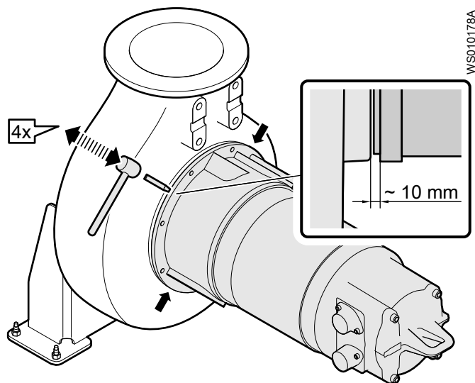
Рис. 85: Демонтаж блока привода
