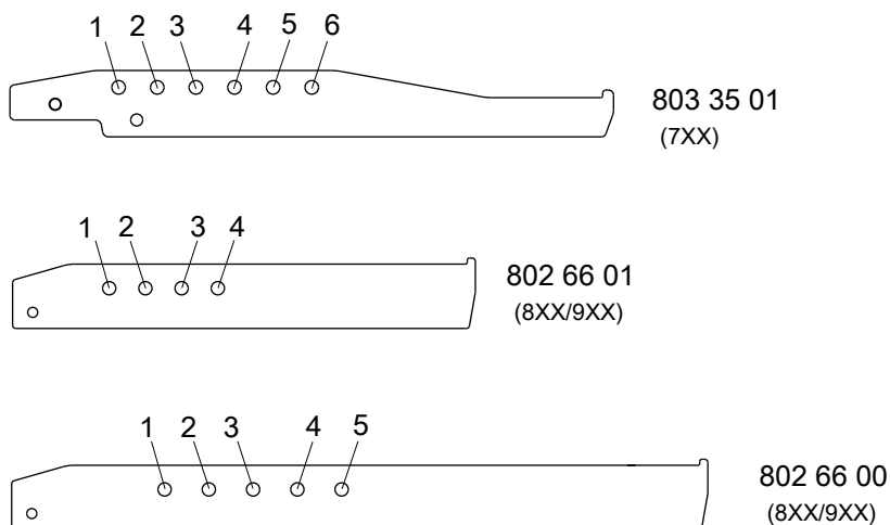
Табл. 33: Положение скобы для подъема привода и рабочего колеса
